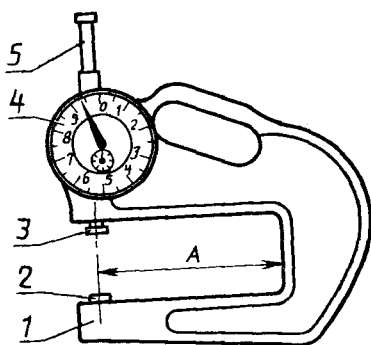
1—корпус; 2—пятка; 3—измерительный наконечник; 4—отсчетное устройство; 5—измерительный стержень; А—вылет
