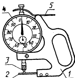
1—корпус; 2—неподвижный стержень; 3—измерительный наконечник; 4—отсчетное устройство; 5—арретир
