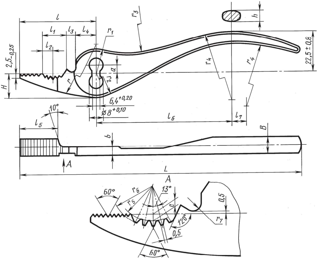
Деталь 2. Рычаг подвижный (черт. 2 и табл. 1)
