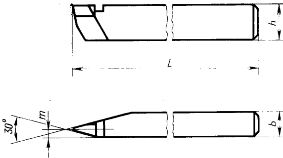
Черт. 3 Размеры в мм
