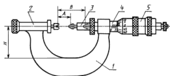
Микрометры типов МВМ, МВТ, МВП
