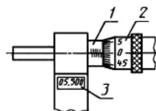
Цифровое устройство микрометров типов МВМЦ, МВТЦ, МВПЦ
