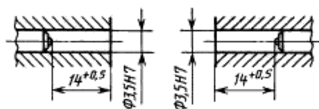
Отверстия под вставки
