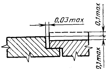
ИСПОЛНЕНИЕ 2
