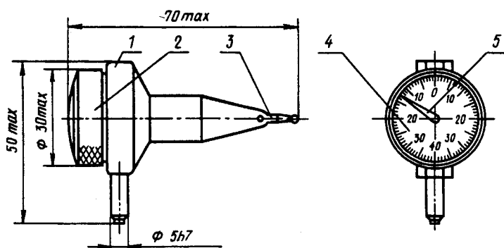
1 — корпус; 2 — ободок; 3 — измерительный рычаг; 4 — циферблат; 5 — стрелка
