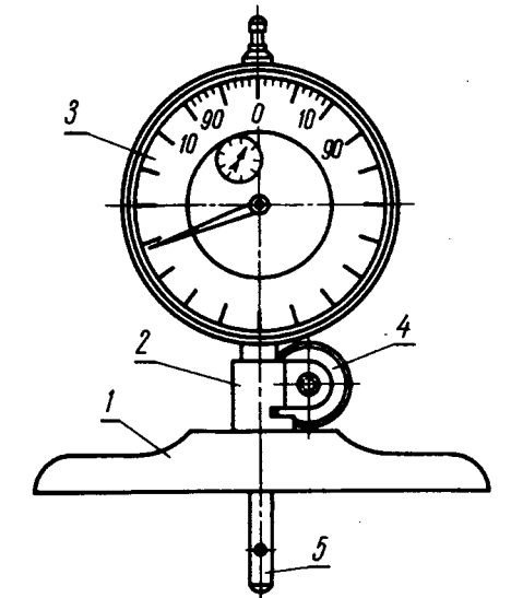
1 — основание; 2 — державка; 3 — индикатор; 4 — винт крепления индикатора; 5 — сменный измерительный стержень
